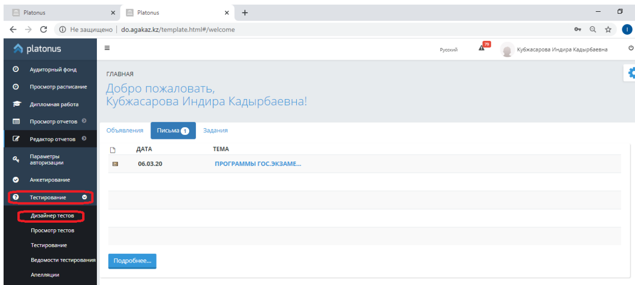
Рис.1. Вкладка «Тестирование»
